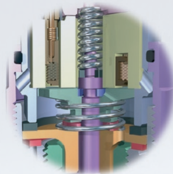
Клапанная группа
