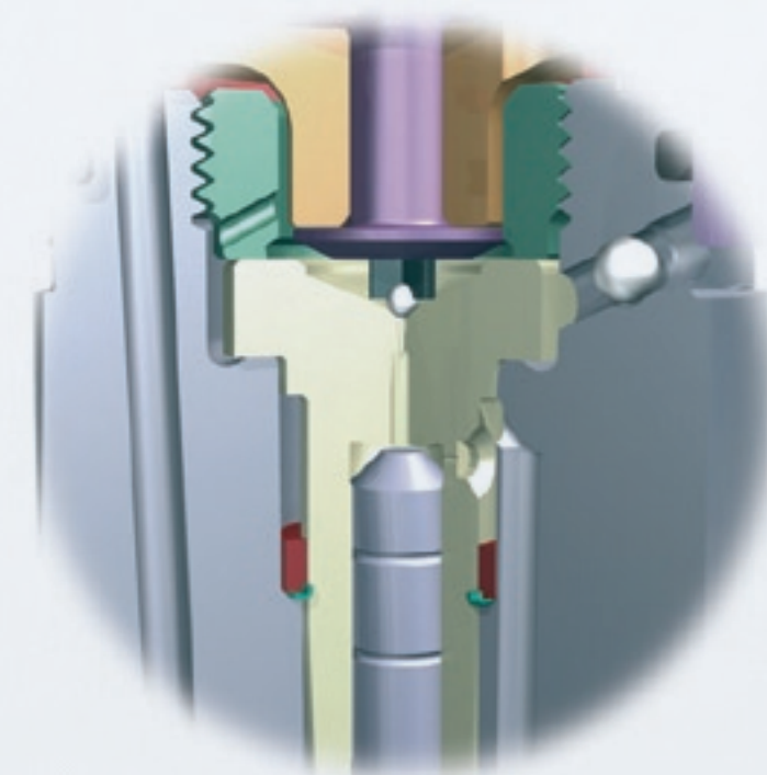
Клапанная группа
